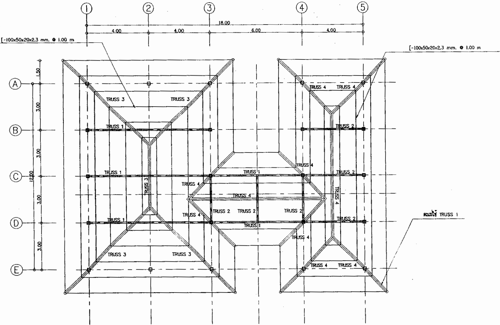
แบบนโครงสร้างหลังคา (TRUSS) มาตราส่วน 1 : 100
