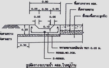
รูปตัดวางระบายน้ำ คสล. โหลปูน
