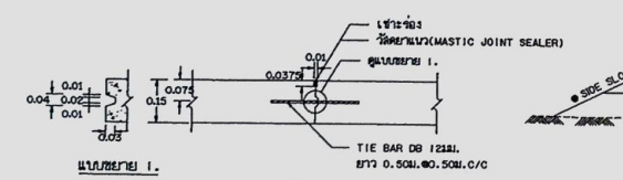
รายละเอียด LONGITUDINAL JOINT
