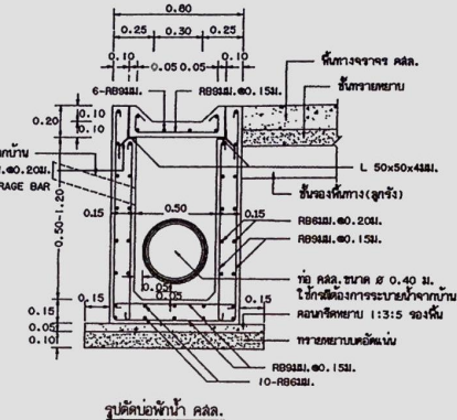
รูปตัดช่องน้ำ คสล.
