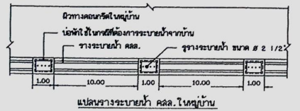
แปลนวางระบายน้ำ คสล. โหลปูน
