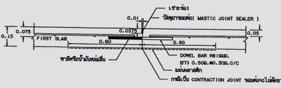
รายละเอียด CONSTRUCTION JOINT และ CONTRACTION JOINT
