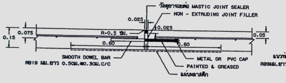
รายละเอียด EXPANSION JOINT
